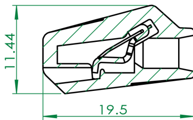
剖面 B-B
